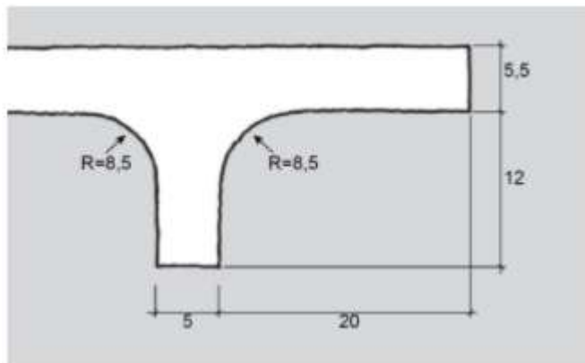
Figur 23: Vendehammer for lastebil iht. Statens vegvesenets håndbok N100.
