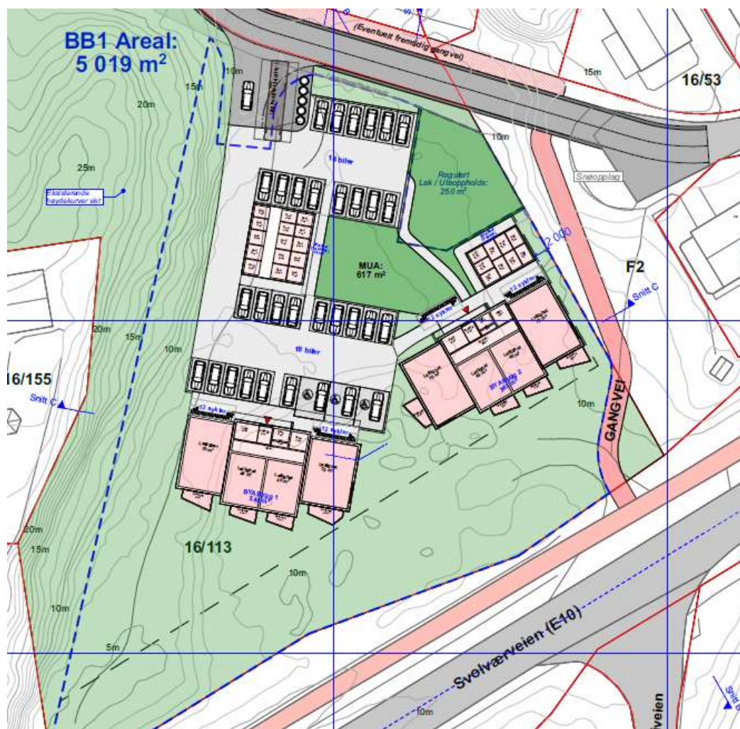
Figur 14. Utsnitt av gjeldende situasjonsplan (alternativ 1). Norconsult.
