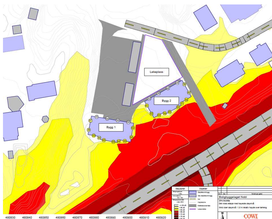
Figur 27. Beregnet støylinje fra veitrafikk, 1,5 meter over bakkeplan. Kilde: Cowi.
