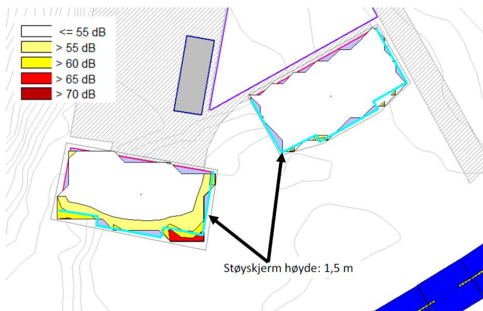
Figur 28. Støysituasjon med 1,5 m høy støyskjerm på takterasser. Støysoner viser støylinje 1,5 m over terrassegulv. Kilde: Cowi.
