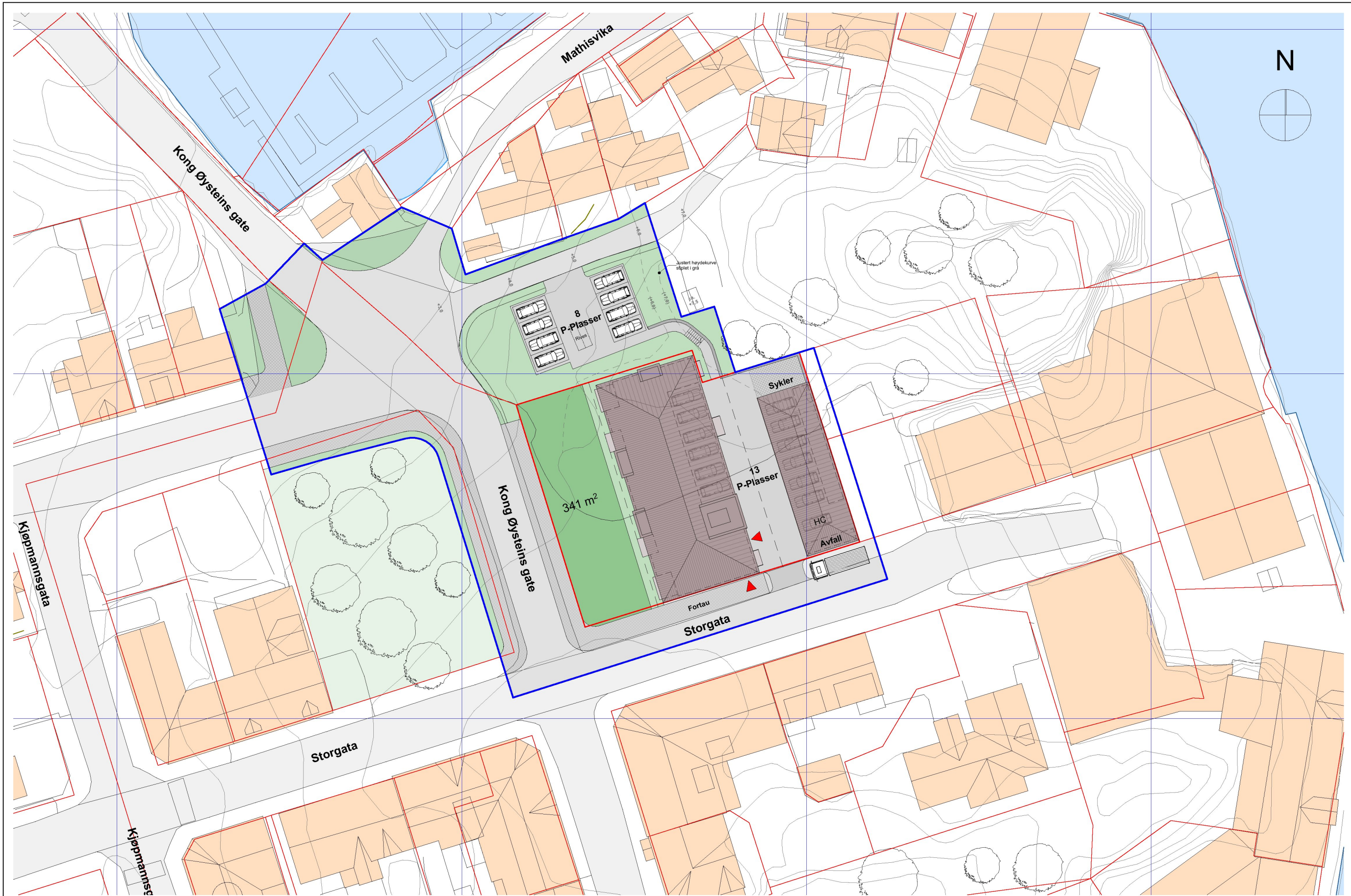
5205878 - A.10.1 - Samlagstomta boliger, Kabelvåg - Situasjonsplan - 2022-10-10 - 1:500
