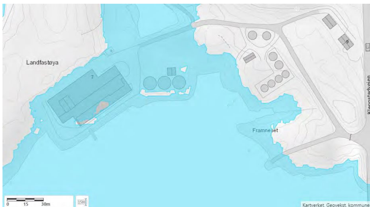
Figur 8: Oversiktskart over naturfarer viser området som påvirkes av stormflo med 200 år gjentakintervall (blått). [Kilde: nve.atlas.no]
