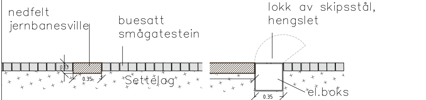
Tverrsnitt tresville
