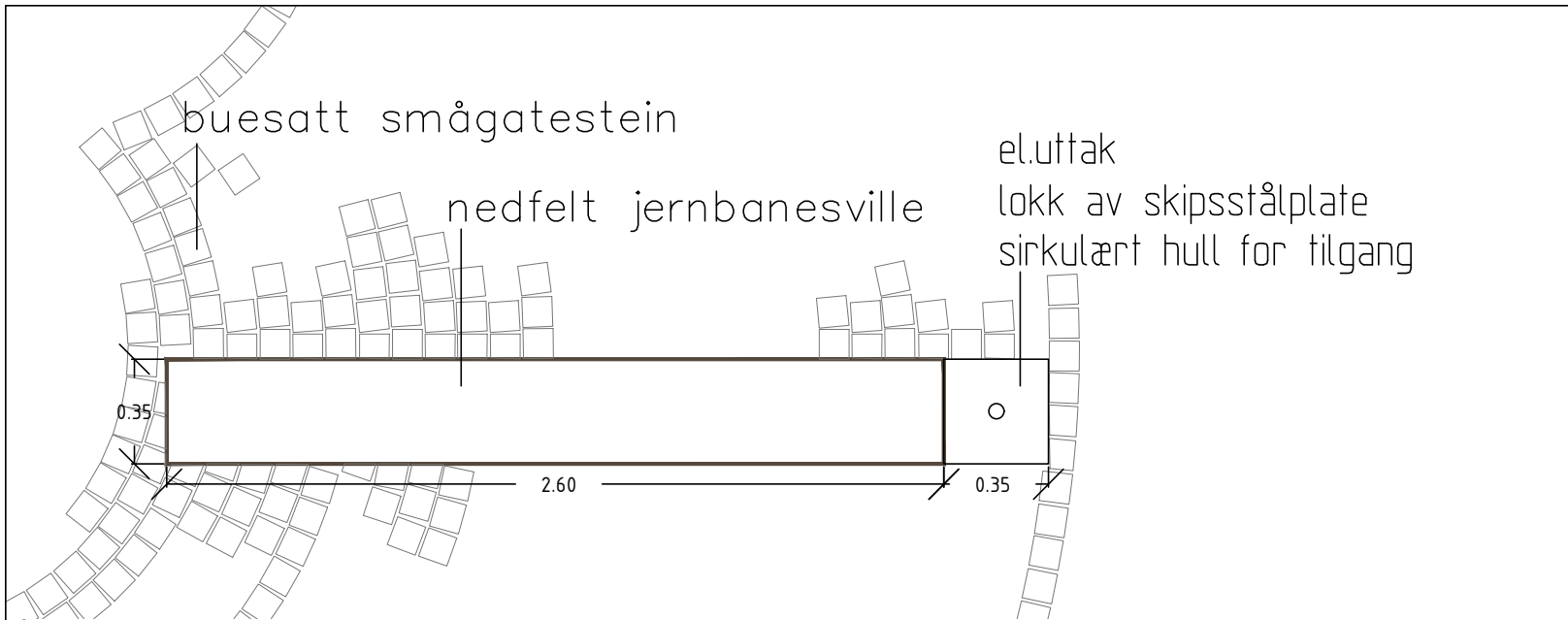
Planutsnitt
