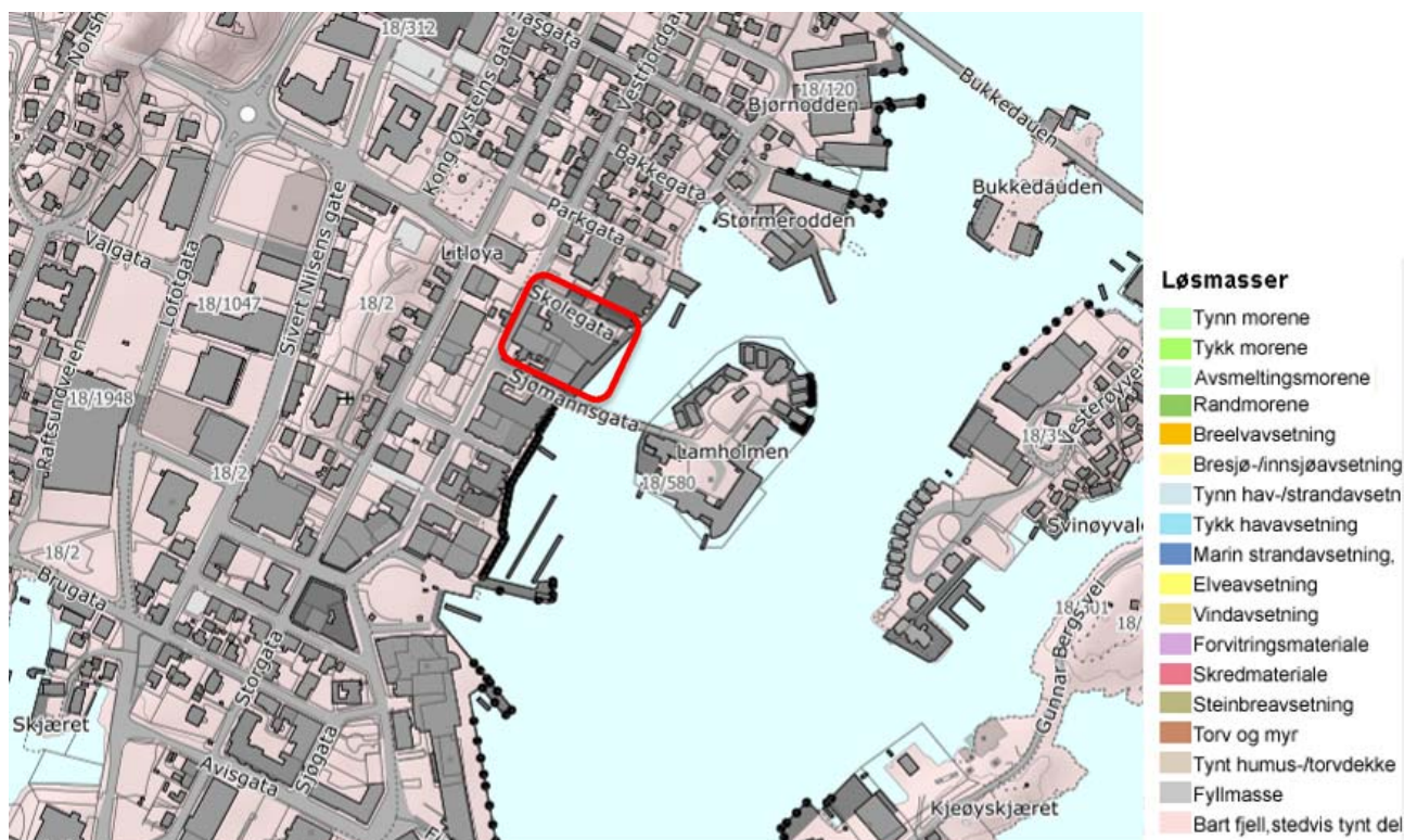
Figur 4-1 Kwartærgeologisk kart over området [5].
